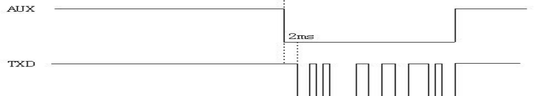
接收模块时序图：
